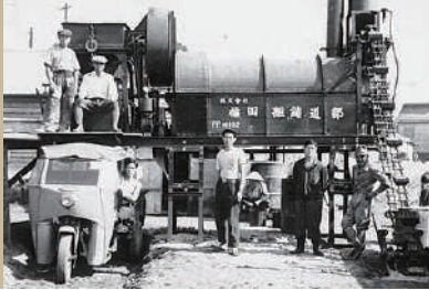
▼1951 舗道部第1号アスファルトプラント
